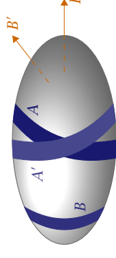
► 9 Die beiden Bahnen A und A' sind Extremalbahnen. Zu ihnen gehören die Magnetfelder B, bzw. B'. Die Bahn B erfüllt die Bedingung für eine Extremalbahn nicht. Nach Hunklinger [2].
