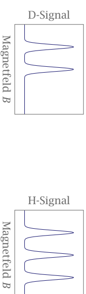
► 71 Die Anzahl der Linien, die im Signal sichtbar sind entspricht der Multiplizität des jeweiligen Kerns.
