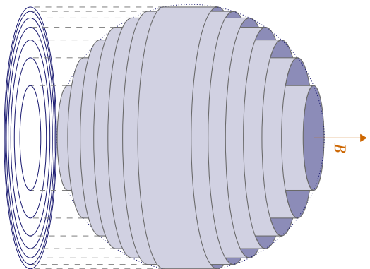
► 12 Die Landau-Röhren des freien Elektronengases werden durch die Fermi-Kugel eingegrenzt. Unterhalb ist die zweidimensionale Projektion abgebildet. Nach Hunklinger [2].
