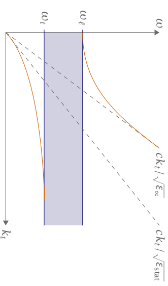
► 87 Dispersionsrelation des Polaritons (orange). Die Dispersionskurven der Phononen verlaufen waagrecht (dunkelblau), die Dispersionskurven des Lichts sind für zwei Grenzfälle eingezeichnet (gestrichelt). Der verbotene Bereich ist hellblau hinterlegt.
